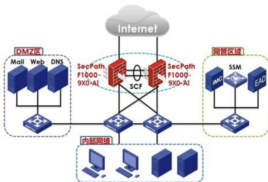
H3C SecPath F1000-9X0-AI 系列组网应用示意图
